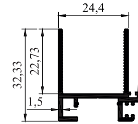
1700-216 SÜRME KENET 0.485 KG/M
