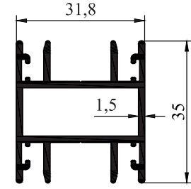
1700-215 SÜRME KENET 0.715 KG/M
