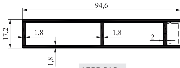
1700-213 YAN KASA 1.135 KG/M
