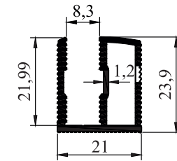
1700-194 BEMUS 8MM U 0.395 KG/M
