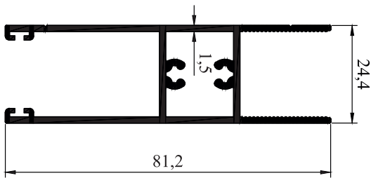
1700-217 SÜRME KANAT 0.970 KG/M
