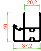
TGI-106 KENET (ISICAM) 0.913 KG/M
